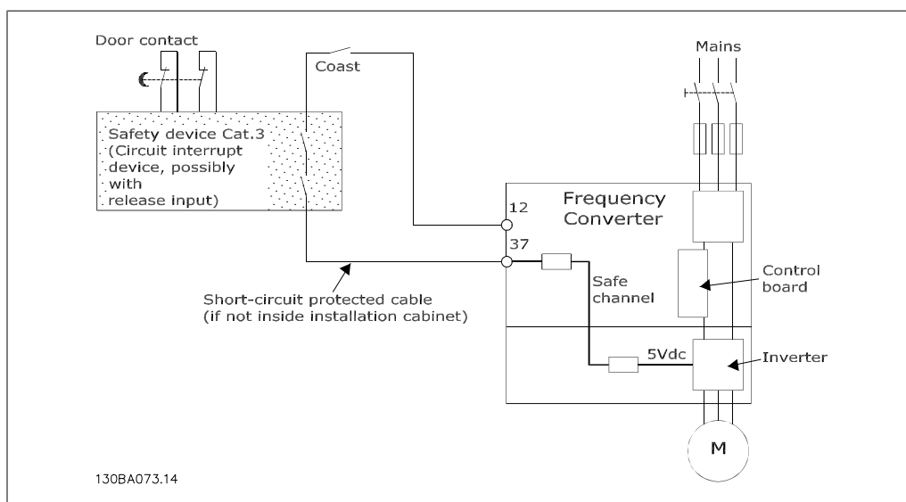
Рисунок 2.5: Рисунок, поясняющий основные особенности установки, необходимые для осуществления останова категории 0 (EN 60204-1), отвечающего требованиям категории безопасности 3 (EN 954-1).
