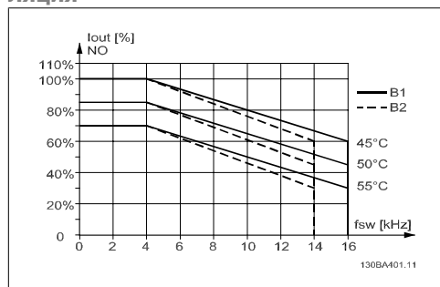
Рисунок 3.5: Снижение тока I_{out} для различных значений T_{AMB, max} для корпуса В при использовании модели коммутации 60 AVM в режиме нормального крутящего момента (перегрузка по крутящему моменту 110 %).
