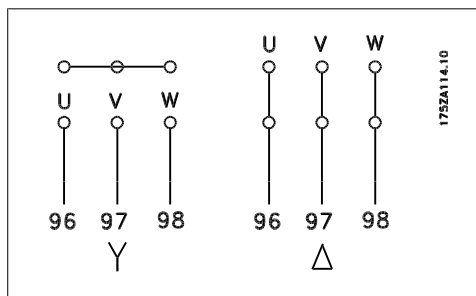
Рисунок 5.11: Подключение двигателя в случае корпусов C1 и C2.
