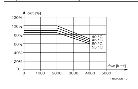
Рисунок 3.16: Снижение тока I_{out} для различных значений T_{AMB, max} для корпуса Е при напряжении 480 В при использовании модели коммутации SFAVM в режиме нормального крутящего момента (перегрузка по крутящему моменту 110 %).
