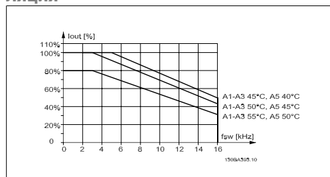
Рисунок 3.1: Снижение тока I_{out} для различных значений T_{AMB, max} при использовании корпуса А и модели коммутации 60 AVM
