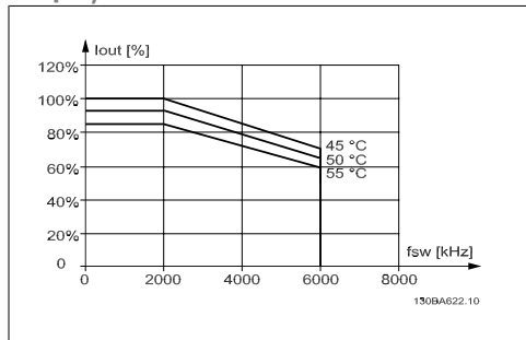
Рисунок 3.15: Снижение тока I_{out} для различных значений T_{AMB, max} для корпуса Е при напряжении 480 В при использовании модели коммутации 60 AVM в режиме нормального крутящего момента (перегрузка по крутящему моменту 110 %).
