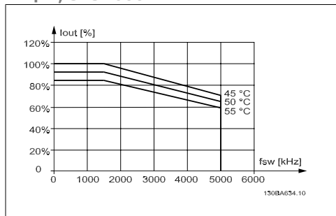
Рисунок 3.17: Снижение тока I_{out} для различных значений T_{AMB, max} для корпуса Е при напряжении 600 В при использовании модели коммутации 60 AVM в режиме нормального крутящего момента (перегрузка по крутящему моменту 110 %).
