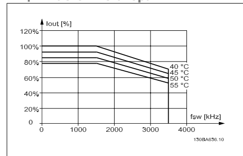
Рисунок 3.18: Снижение тока I_{out} для различных значений T_{AMB, max} для корпуса Е при напряжении 600 В при использовании модели коммутации SFAVM в режиме нормального крутящего момента (перегрузка по крутящему моменту 110 %).
