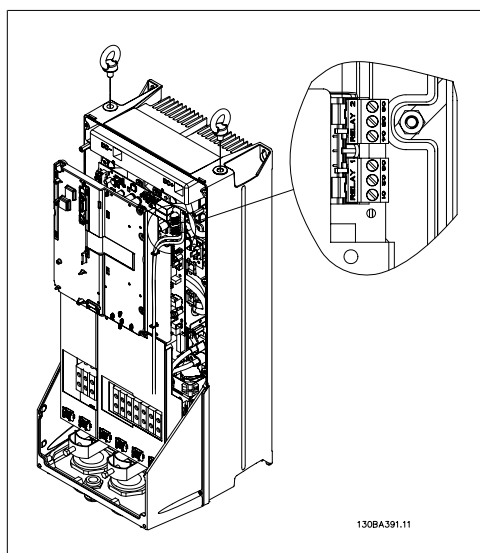
Рисунок 5.19: Клеммы для подключения реле
