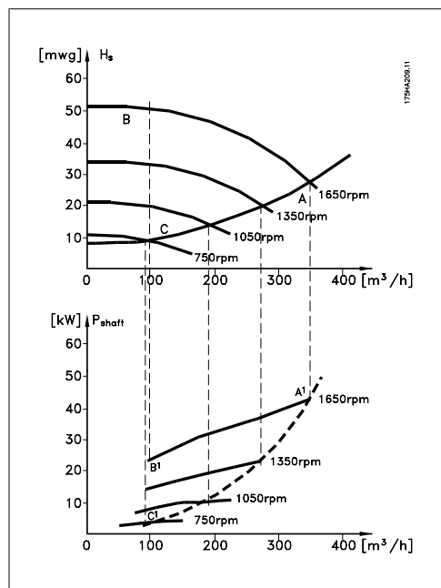
Характеристики насоса
