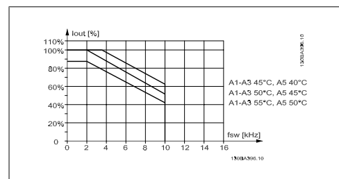
Рисунок 3.4: Снижение тока I_{out} для различных значений T_{AMB, MAX} в случае корпуса А, при использовании модели коммутации SFAVM и длине кабеля до 10 м.
