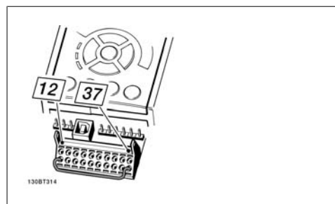
Рисунок 5.17: Перемычка между клеммой 37 и источником напряжением 24 В=.
