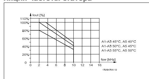
Рисунок 3.2: Снижение тока I_{out} для различных значений T_{AMB, MAX} в случае корпуса А при использовании модели коммутации 60 SFAVM
