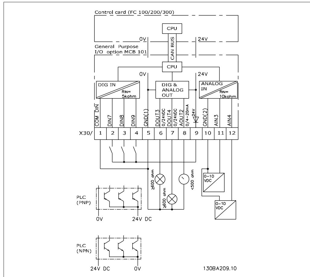
Рисунок 3.10: Принципиальная схема
