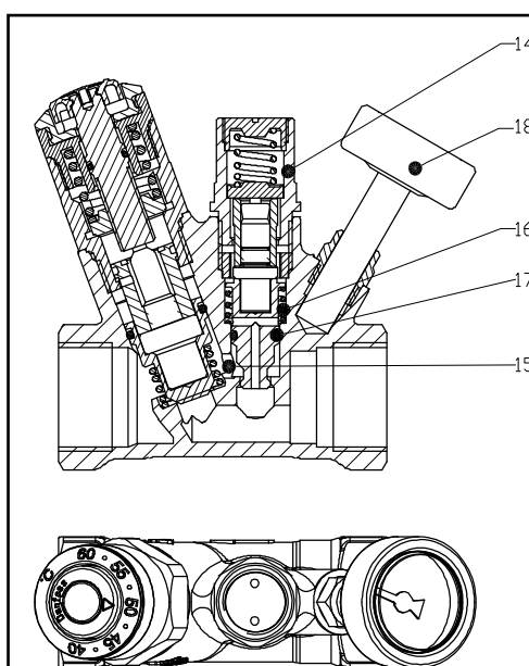
Рис. 6. Версия клапана MTCV с функцией автоматической дезинфекции системы горячего водоснабжения - «В»*
